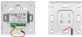
Рис. 7. Подключение датчика температуры воздуха
