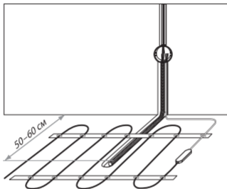
Рис. 3. Монтаж терморегулятора и нагревательной секции
