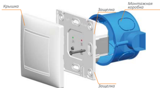
Рис. 8. Схема сборки-разборки терморегулятора
