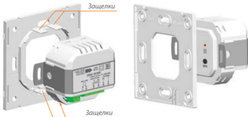
Рис. 9. Демонтаж съёмной рамки
