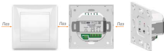
Рис. 6. Снятие крышки прибора
