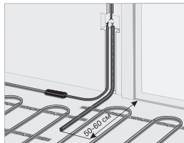
Рис. 8 Монтаж датчика температуры пола
