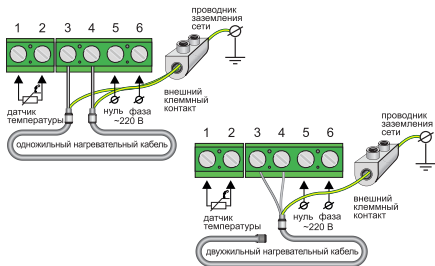
Рис.10 Схема подключения терморегулятора к 3-х проводной электросети
