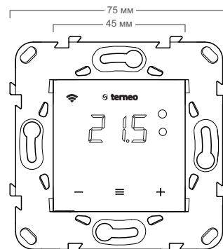
Рисунок 1. Габаритные размеры
