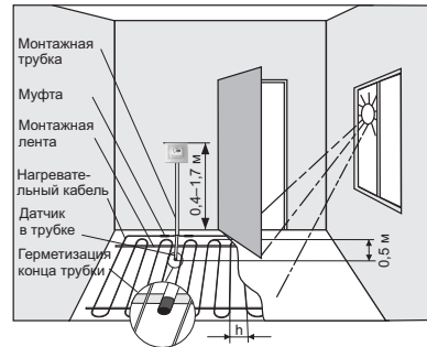
Рисунок 2. Монтаж терморегулятора и теплого пола
