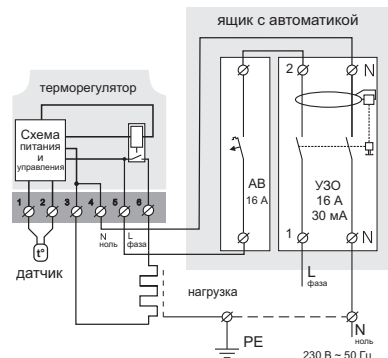
Схема 2. Подключение автоматического выключателя и УЗО
