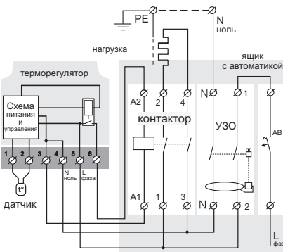
Схема 3. Подключение через контактор
