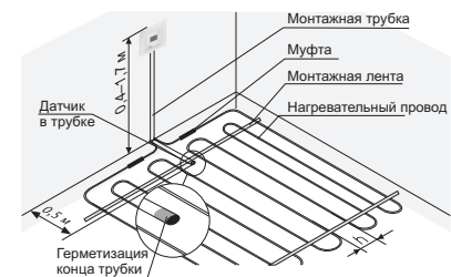
Рисунок 1. Монтаж терморегулятора и теплого пола
