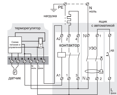
Схема 3. Подключение через контактор
