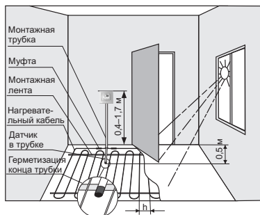
Рисунок 1. Монтаж терморегулятора и системы теплых полов
