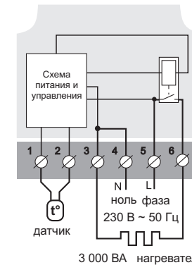
Схема 1. Схема подключения и упрощенная внутренняя схема
