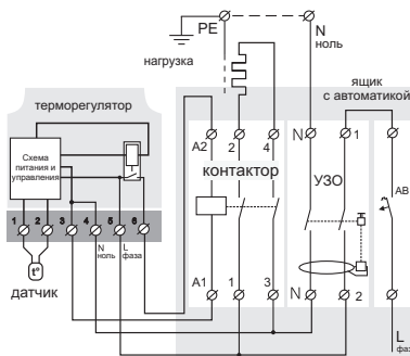
Схема 3. Подключение через контактор
