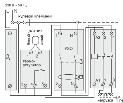
Схема 3. Подключение через магнитный пускатель
