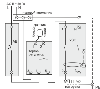
Схема 2. Подключение АВ и УЗО
