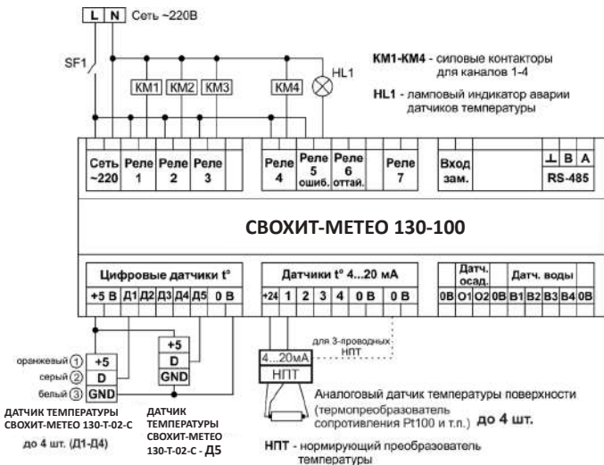
Рисунок 11. Схема подключения СВОХИТ-МЕТЕО 130-100 в режиме «Труба+»
