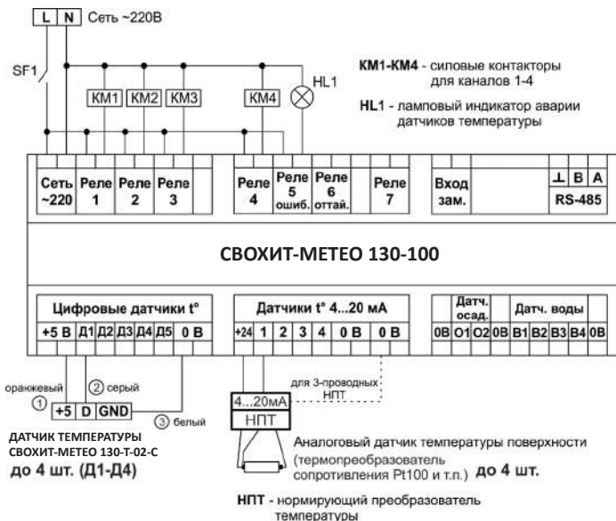
Рисунок 8. Схема подключения СВОХИТ-МЕТЕО 130-100 в режиме «Труба»
