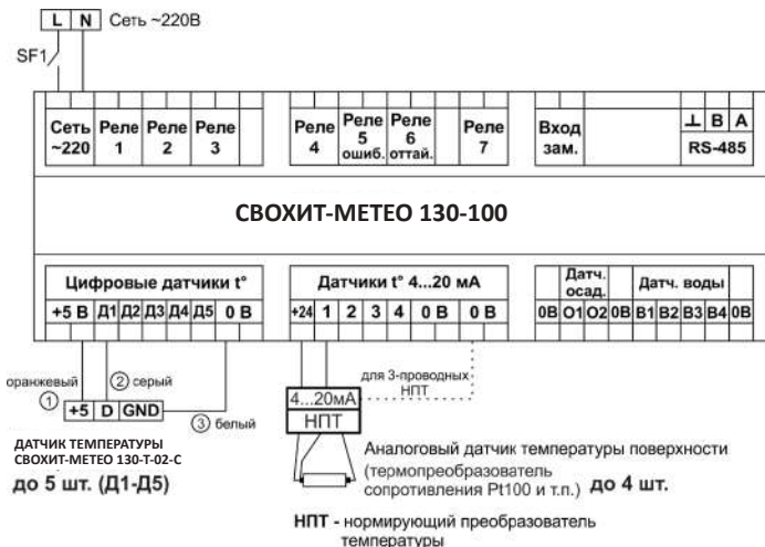
Рисунок 23. Схема подключения СВОХИТ-МЕТЕО 130-100 в режиме «t датчиков»
