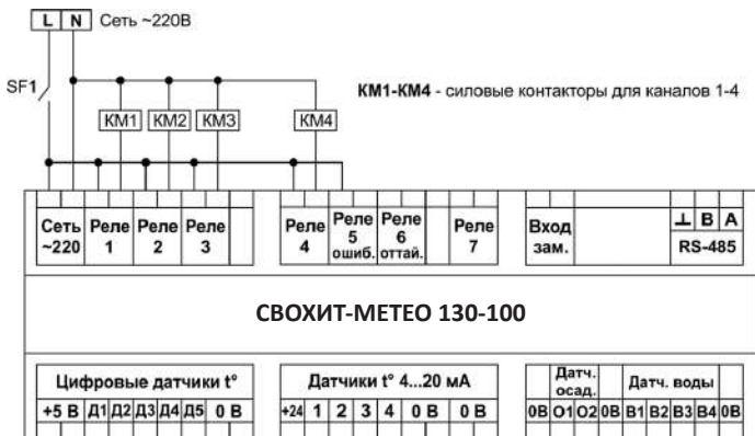
Рисунок 19. Схема подключения СВОХИТ-МЕТЕО 130-100 в режиме «Таймер»
