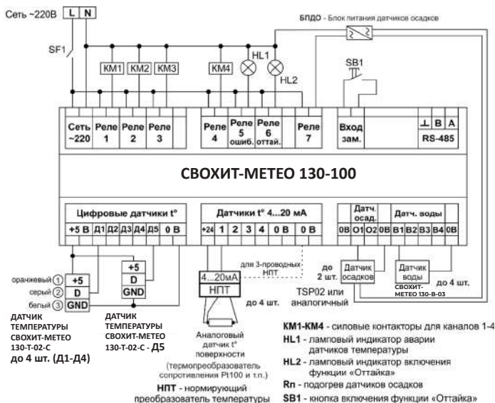
Рисунок 15. Схема подключения СВОХИТ-МЕТЕО 130-100 в режиме «Кровля/дор»
